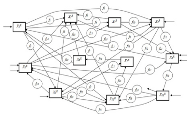
Рис. 1. Ориентированный граф взаимосвязей между X1R(t) - X11R(t)
